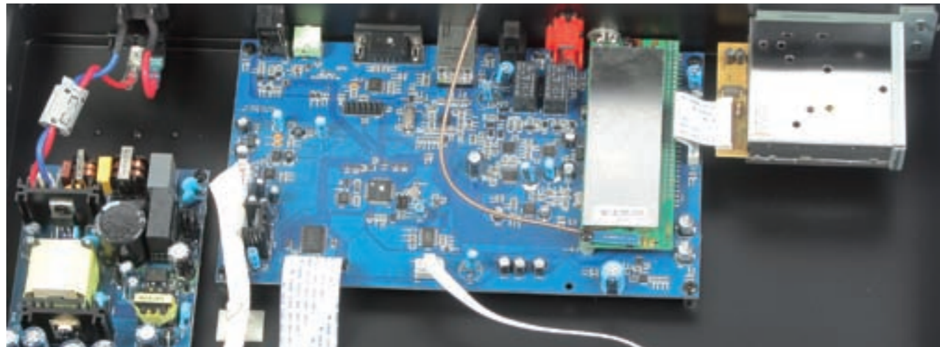
BEIM JUPITER: Unter der Abschirmhaube am rechten Rand der Hauptplatine verbirgt sich der Jupiter6-Chipsatz von Frontier Silicon, der Streaming, Internetradio und DAB auf einem Board vereint. Ganz rechts das durchaus seriöse Analogtuner-Modul, am linken Bildrand das Schaltnetzteil. Die Audioabteilung mit Burr-Brown-Wandler und Ausgangsstufen befindet sich links neben dem Streaming-Hangar.
